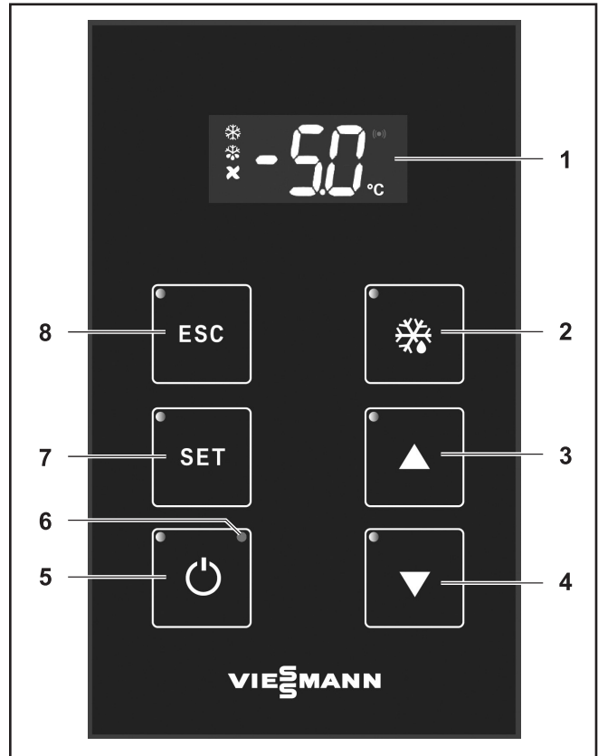
Abbildung 1: Bedienelement
